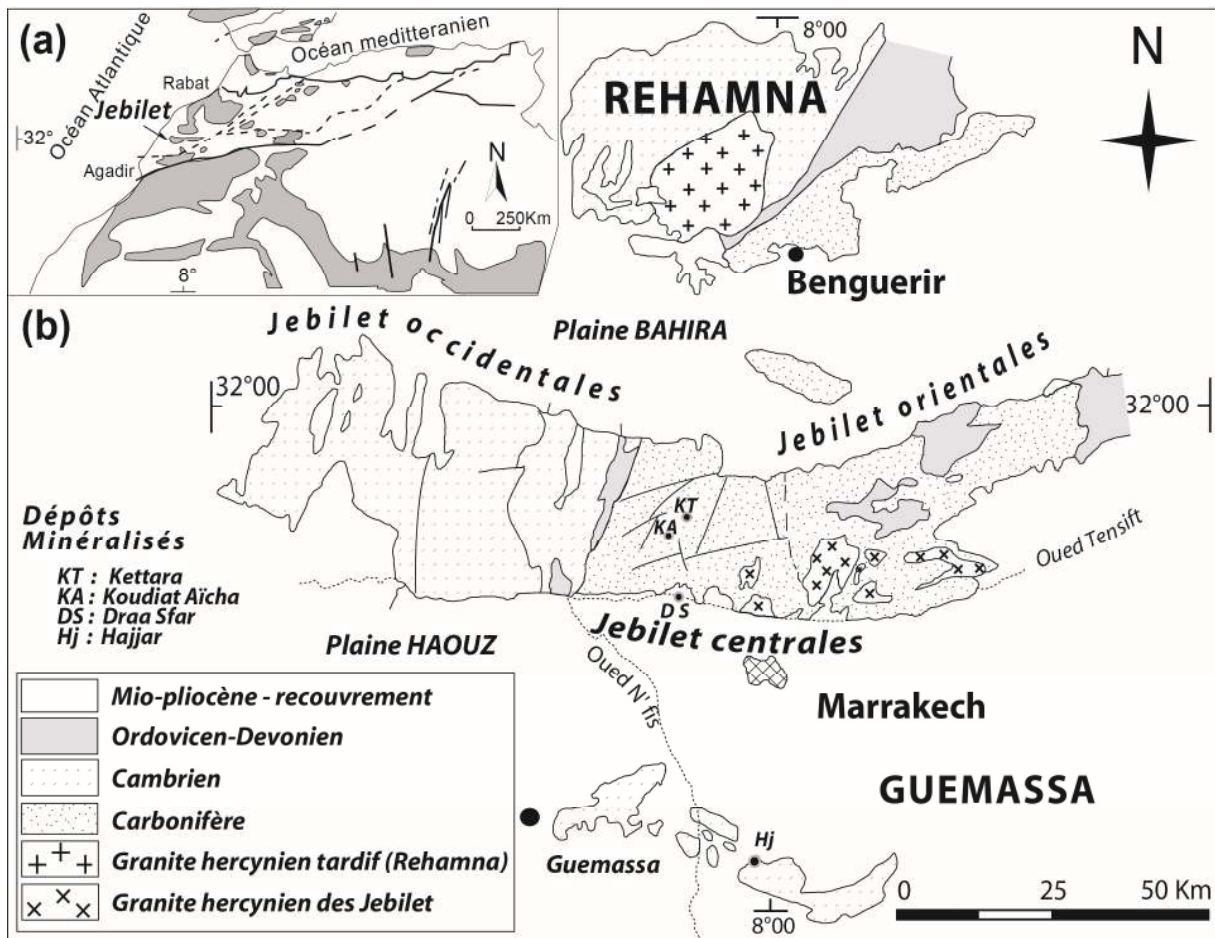
Fig. 1. (a) Situation géographique du massif des Jebilet dans le Maroc hercynien, (b) Esquisse géologique des massifs hercyniens du Maroc : Rehamna, Jebilet et Guemassa
