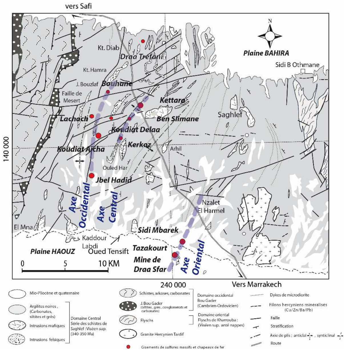
Fig. 2. Carte géologique simplifiée des Jebilet centrales et localisations des chapeaux de fer (Huvelin, 1977)
