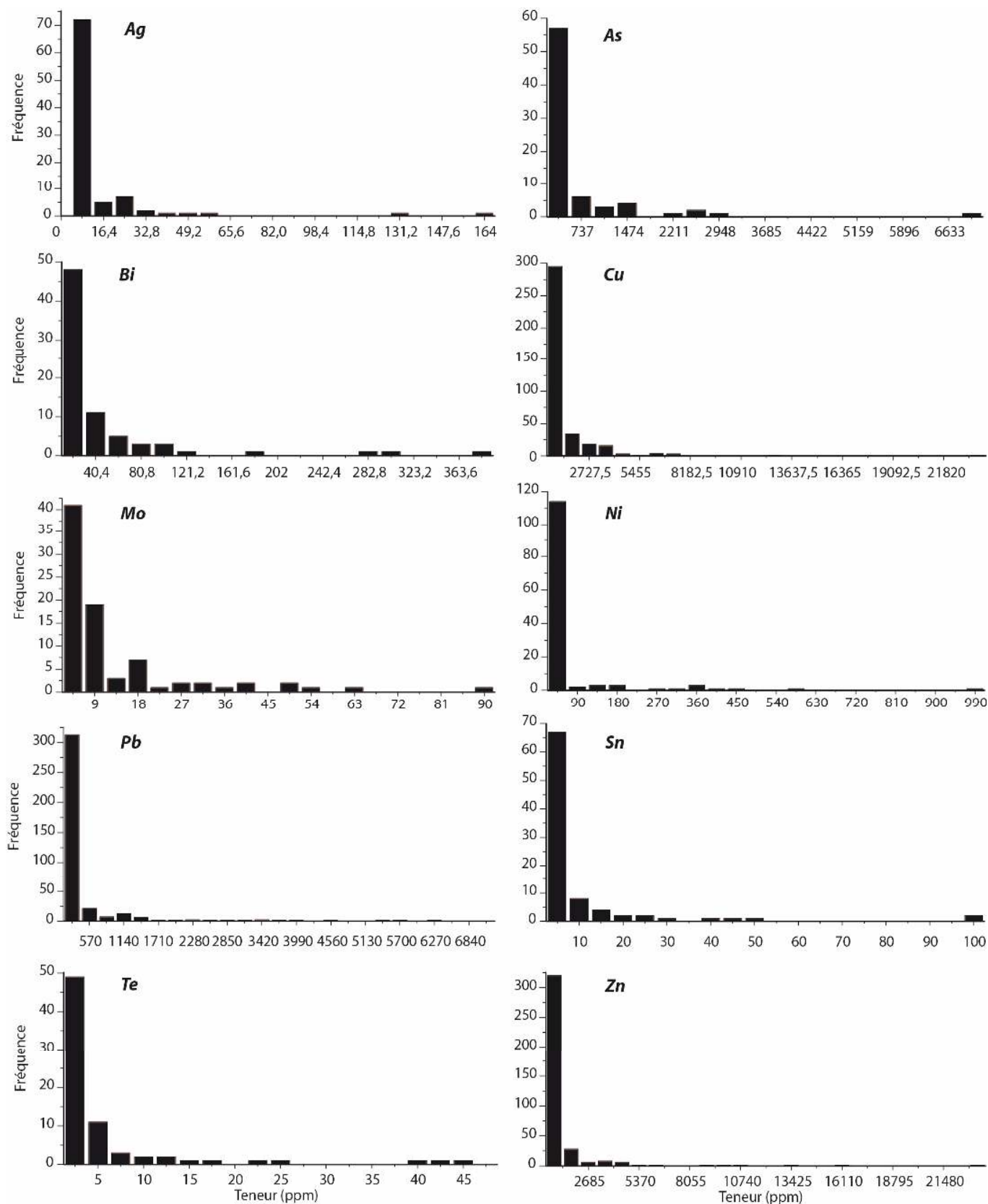
Fig. 3. Histogramme de fréquence des éléments traces des chapeaux de fer des Jebilets centrales
